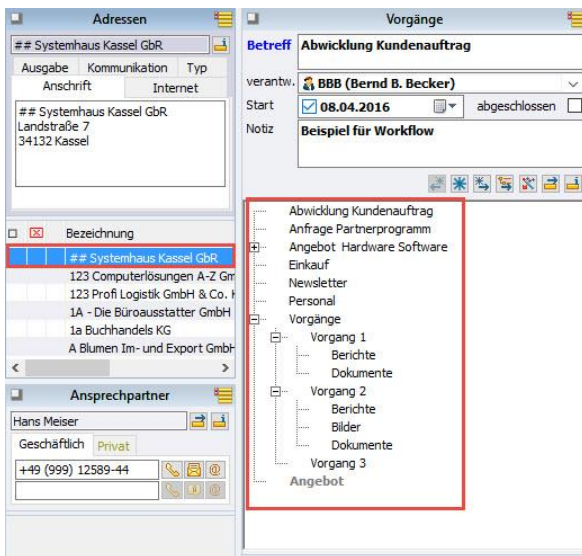
Screenshot alle Vorgänge einer Adresse
